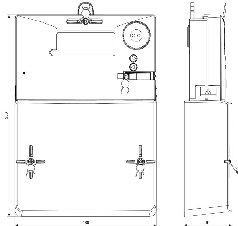
LEPUS mit Standard-Klemmkastendeckel
