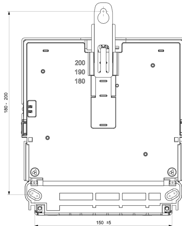
Befestigungslöcher LEPUS
